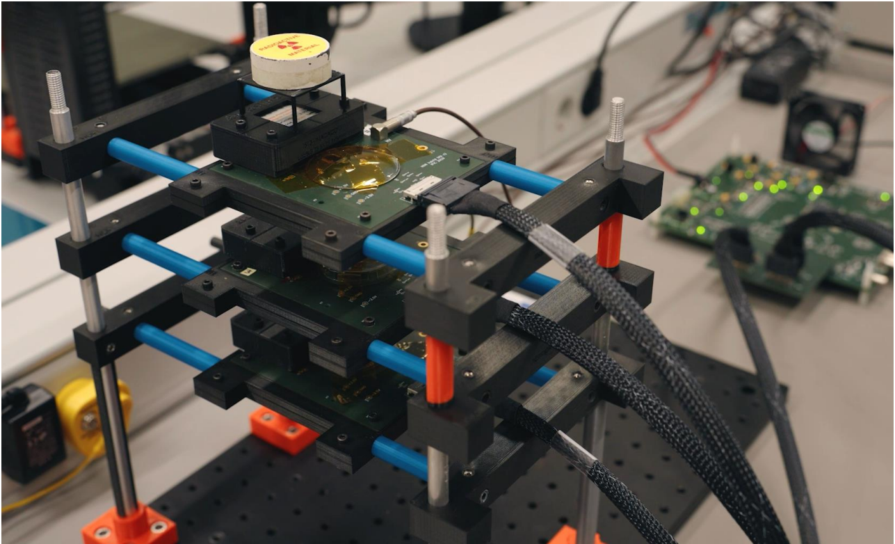
Imagen 1. Dispositivo de detección ensamblado en el laboratorio.
