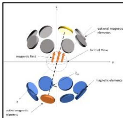
Imagen 2. Imagen esquemática del funcionamiento del dispositivo.
