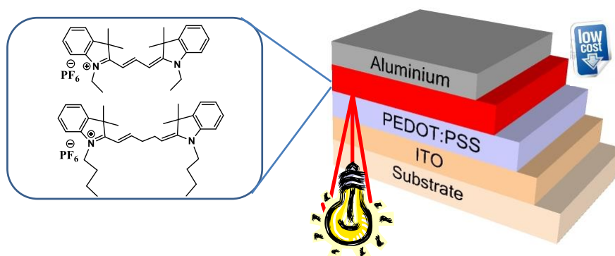
Imagen 1: Esquema del dispositivo y ejemplos de tintes cianúricos usados como material activo
